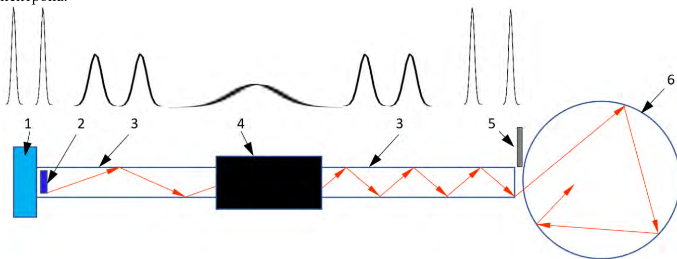
Рис. 24. Идея источника УХН для импульсного источника с использованием временной фокусировки. 1 – замедлитель, 2 – конвертер УХН, 3 – зеркальный нейтронотвод, 4 – фокусирующее устройство, 5 – быстрый затвор, 6 – ловушка УХН
