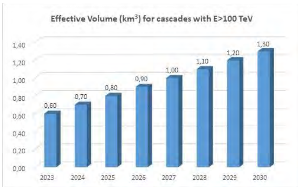
Рис. 11. Эксперимент Ваикал-GVD. План расширения детектора в терминах эффективного объема в задаче регистрации астрофизического потока
