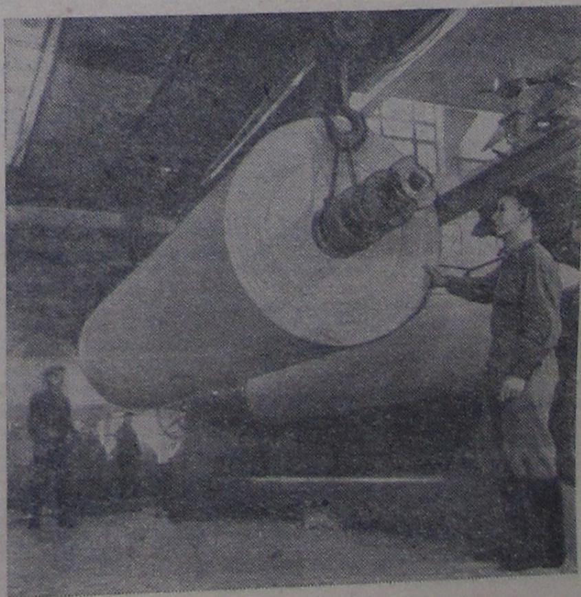
Красноярск. На целлюлозно-бумажном комбинате введена в действие первая в Сибири технологическая линия по производству газетной бумаги. По мощности нет равных в стране. С бумагоделательной машины ежесекундно снимается бумажная лента длиной в 30 километров и шириной более четырех метров.
