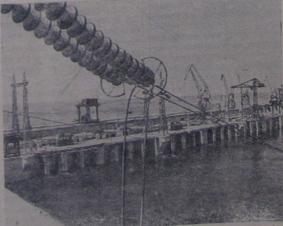
На снимке: вид на Кременчугскую ГЭС с нижнего бьефа.
