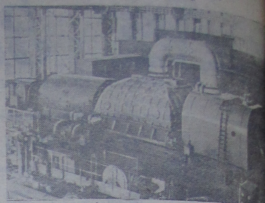
На снимке: турбогенератор № 1 Назаровской ГРЭС мощностью 150 тысяч киловатт, который недавно вступил в строй. Фото Ю. БАРИНА.
