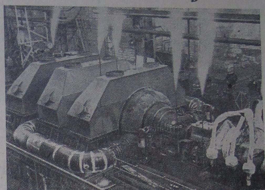
Большую трудовую победу одержал коллектив Ленинградского Металлического завода — закончена сборка и успешно проведены испытания паровой однофазной турбины мощностью 300 тысяч киловатт. Это новый вклад ленинградских турбостроителей в семилетку.
