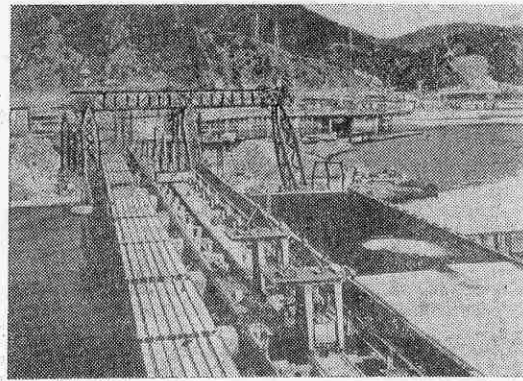
На снимке: строительство гидроэлектростанции «Днердап», которую совместно сооружают на Дунае в районе Железных ворот социалистическая Югославия и Румыния при техническом содействии Советского Союза. После окончания строительства общая мощность этой электростанции составит 2100 тысяч киловатт.
