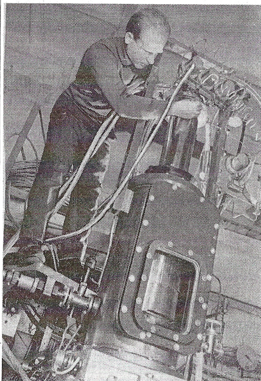
В криогенном отделе Лаборатории высоких энергий была разработана струйная водородная мишень для изучения р-р взаимодействия в внутреннем пучке ускорителя.
