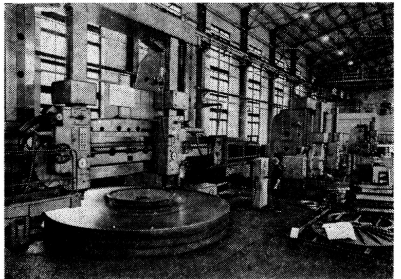
На снимке: механический участок цеха № 2 Центральных экспериментальных мастерских. Здесь производится обработка деталей ускорителя У-120М для ЧССР.
