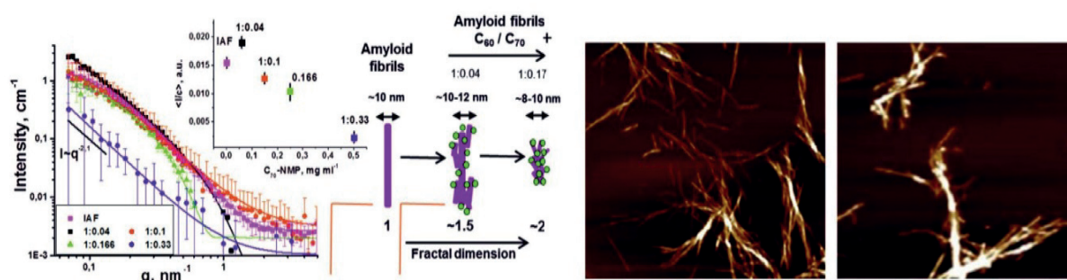
Рис. 2. Изменения в модельных амилоидных растворах лизоцима и инсулина при добавлении фуллеренов по результатам структурных исследований, в том числе методами МУРН и АСМ.
