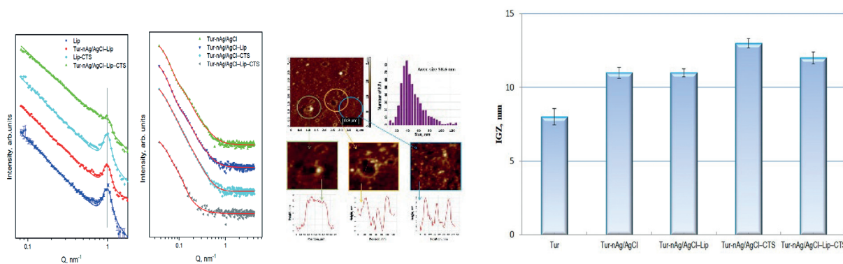
Рис. 2. Структурно-морфологические характеристики биогридов (слева направо: SANS, SAXS и AFM) и их антибактериальный эффект на Enterococcus faecalis .
