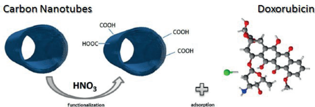
Рис. 1. Схема модификации углеродных нанотрубок и адсорбции на них доксорубицина.
