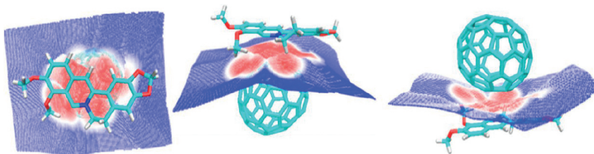
Рис. 2. Расчетные электронные плотности при возможном комплексообразовании фуллерена C70 и противоракового препарата на основе берберина.
