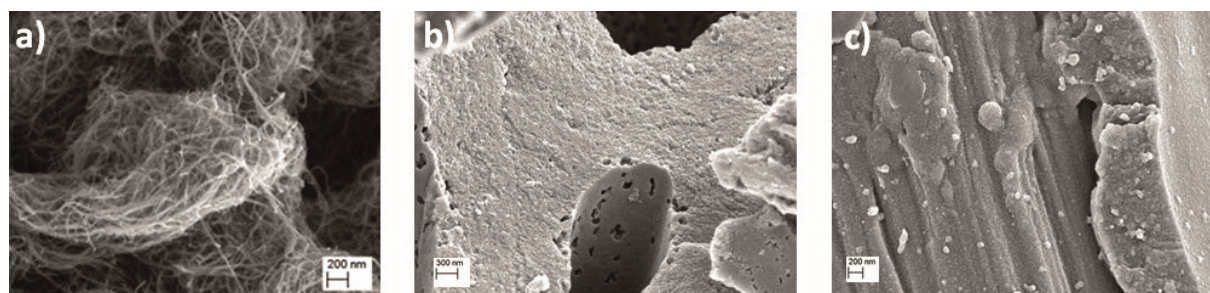
Рис. 2. Изображения со сканирующего электронного микроскопа (SEM) модифицированных а) углеродных нанотрубок и б) активированного угля, а также с) углеродных волокон с адсорбированным доксорубицином.
