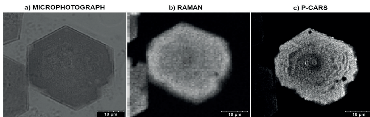
Рис. 1. Визуализация кристалла бР: микрофотография (а), рамановская спектроскопия (б), П-КАРС (с).
