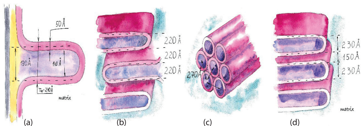
Рис. 2. Строение кристы митохондрии печени в условиях (а) набухания матрицы (гипотонических условиях) и кристы митохондрий сердца в (b) нормальных (изотонических) условиях и (c, d) гипотонических условиях.
