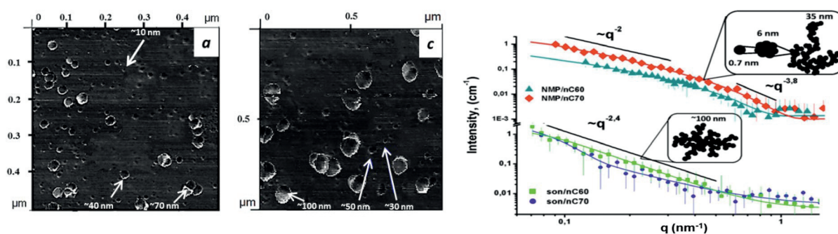
Рис. 1. Структура биологически активных растворов фуллеренов C 60 и C 70 по данным атомно-силовой микроскопии и малоуглового рассеяния нейтронов.
