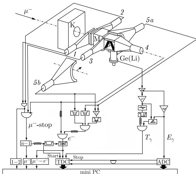
Рис. 22. Блок-схема экспериментальной установки MEGA
