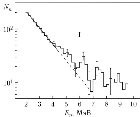
Рис. 17. Энергетический спектр нейтронов из реакции \mu^- -захвата в йоде
