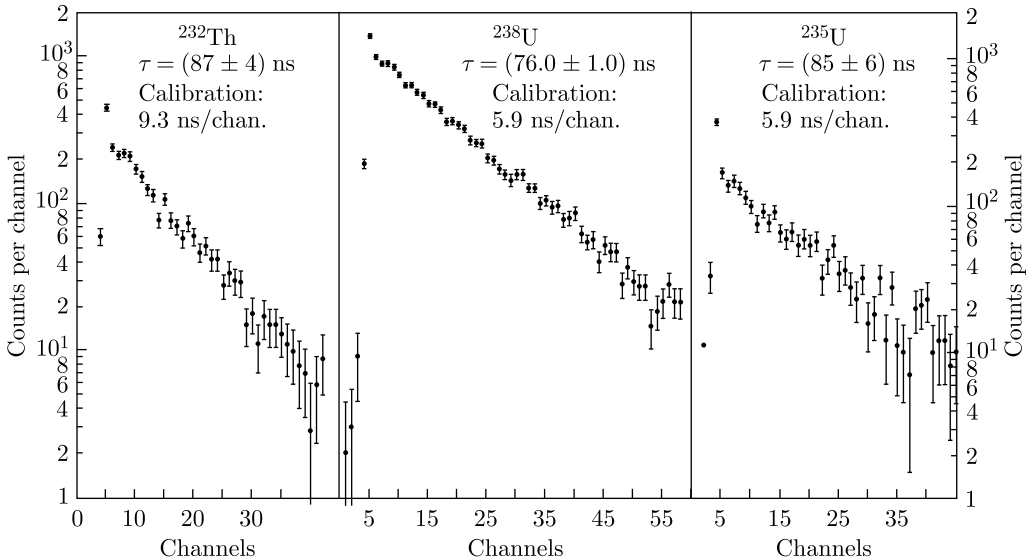
Рис. 8. Временное распределение событий деления в ^{232}\text{Th} , ^{238}\text{U} и ^{235}\text{U} , индуцированных \mu^- -мезонами (фон вычтен)
