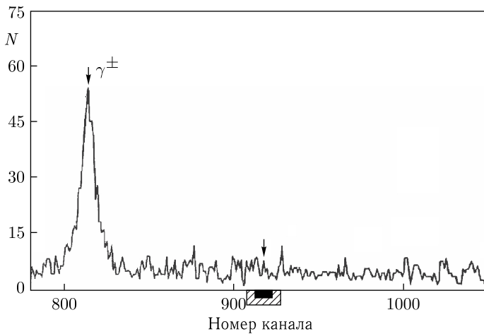
Рис. 24. Спектр задержанных \gamma -квантов с отбором по признаку наличия быстрого электрона от распада мюона. Стрелки указывают положения пиков; темная область — ширина пика на полувысоте, заштрихованная — на 0,1 высоты
