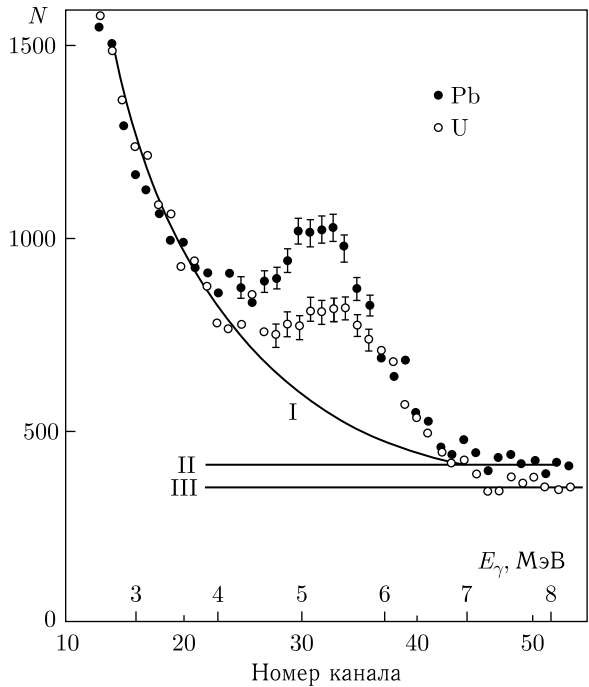
Рис. 2. Спектры фотонов для мезоурана и мезосвинца: I — интерполяция спектров урана и свинца; II — уровень фона, обусловленный интерполяцией спектров урана и свинца; III — грубая оценка фона, полученная в предположении одинаковости ширинок пиков урана и свинца
