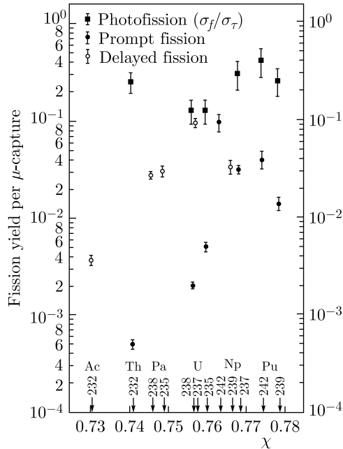
Рис. 10. Абсолютный выход для мгновенного и задержанного деления, вызванного \mu^- -захватом, как функция параметра делимости \chi [32]
