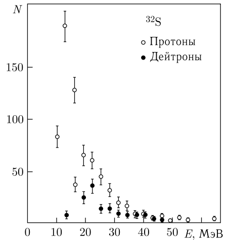
Рис. 20. Энергетический спектр протонов и дейтронов при захвате мюонов ядром ^{32}\text{S} [68]
