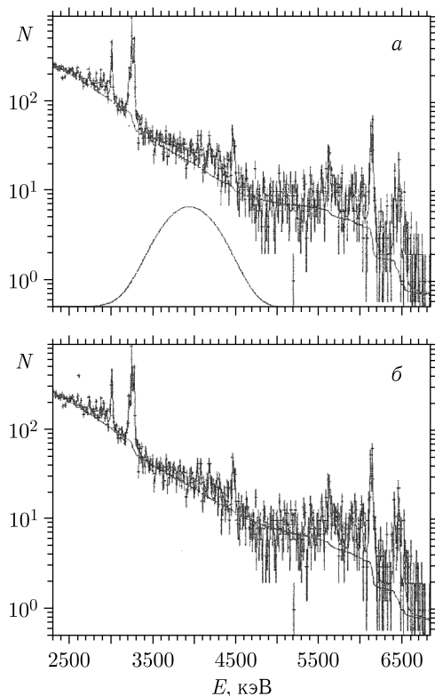
Рис. 5. Спектр мюонного X-излучения, зарегистрированный одним Ge-детектором в совпадении с МД в эксперименте ^{238}\text{U}(\mu^-, \gamma f) [23]. Сплошные линии — подгонка к этому спектру, фон и гауссова кривая. Верхний спектр (а) содержит подгонку с широкой гауссовой структурой при 3910 кэВ, нижний (б) — без такой структуры
