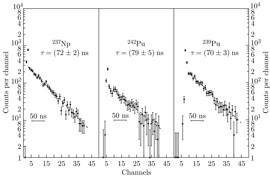
Рис. 9. Временное распределение событий деления в ^{237}\text{Np} , ^{242}\text{Pu} и ^{239}\text{Pu} , индуцированных \mu^- -мезонами (фон вычтен). Линии указывают на соответствие экспоненциальной кривой распада точкам данных. Калибровка: 6,84, 5,8 и 6,14 нс/канал для ^{237}\text{Np} , ^{242}\text{Pu} и ^{239}\text{Pu} соответственно
