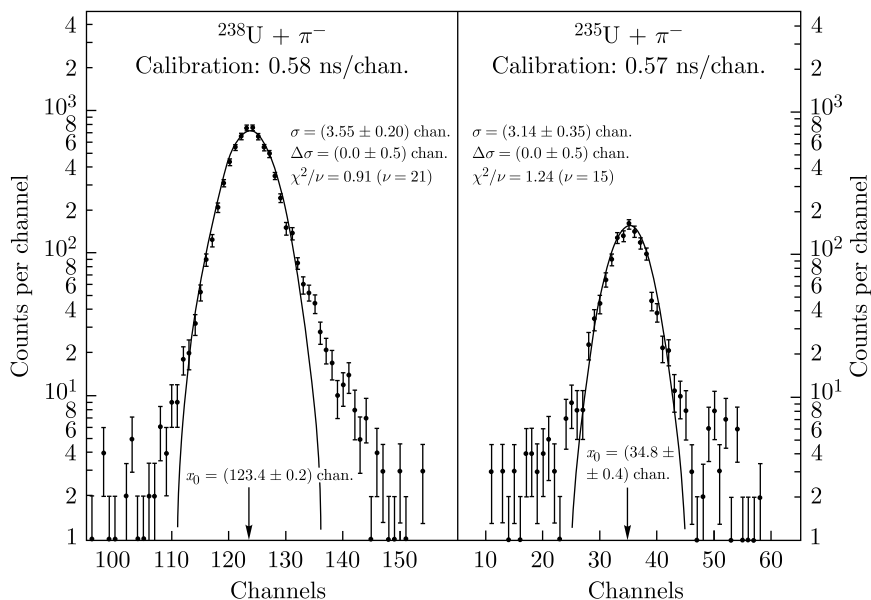
Рис. 7. Примеры временного распределения деления, индуцированного \pi^- -мезонами
