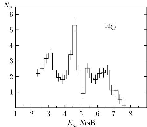
Рис. 15. Энергетический спектр нейтронов из реакции \mu^- -захвата в кислороде
