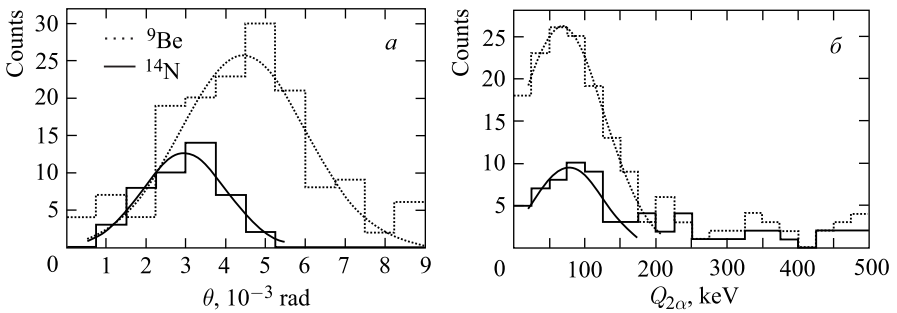
Рис. 3. Распределения углов разлета \theta в парах \alpha -частиц (а) и инвариантной массы Q_{2\alpha} (б) для событий фрагментации ^9\text{Be} \rightarrow ^8\text{Be}_{\text{gs}} при 2A ГэВ/с и ^{14}\text{N} \rightarrow ^8\text{Be}_{\text{gs}} при 2,9A ГэВ/с
