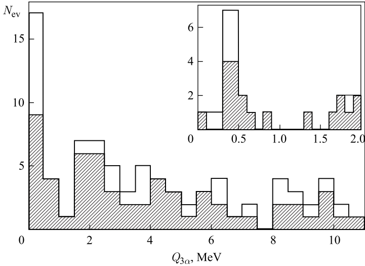
Рис. 6. Распределение по инвариантной массе \alpha -троек Q_{3\alpha} в диссоциации ^{12}\text{C} \rightarrow 3\alpha при импульсе 4,5А ГэВ/с (заштрихованная область) и 1А ГэВ/с (светлая область); на вставке: область по Q_{2\alpha} до 2 МэВ
