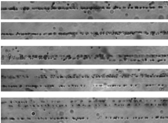
Рис. 2. Фотографии участков события когерентной диссоциации в ЯЭ {}^{12}\text{C} \rightarrow 3\text{He} при 1А ГэВ/с (сверху вниз); при смещении от вершины вдоль струи фрагментов можно различить три фрагмента He
