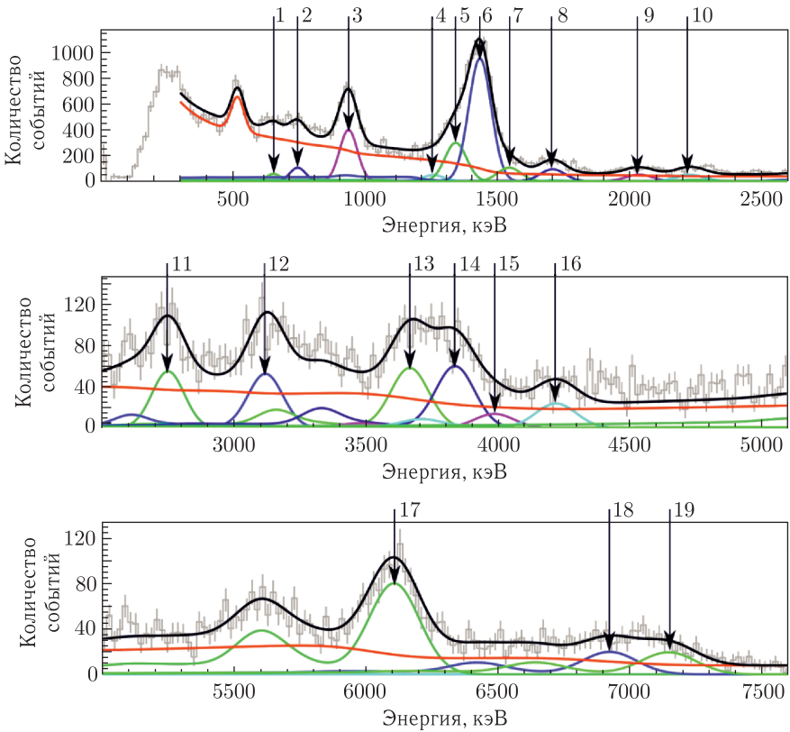
Рис. 18. Применение функции отклика для подгонки энергетического спектра образца оксида хрома, полученного с помощью VGO-детектора под углом \sim 33^\circ к меченому нейтронному пучку. Стрелками указаны положения фотопиков для характеристических \gamma -линий
