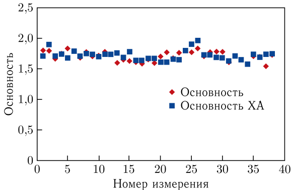
Рис. 37 (цветной в электронной версии). Результаты химического анализа (синие квадраты) в сравнении с результатами анализатора АГП-К-1 (красные ромбы). Каждая точка на графике соответствует усреднению результатов в течение 2 ч
