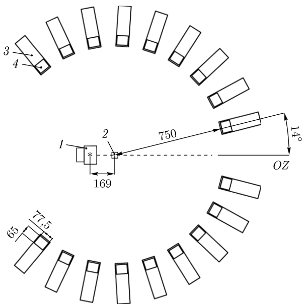
Рис. 16. Схема экспериментальной установки с детекторной системой «Ромаша»: 1 — нейтронный генератор ИНГ-27; 2 — мишень; 3 — \gamma -детектор, входящий в массив из 18 \gamma -детекторов на основе ВГО «Ромаша»; 4 — кристалл ВГО. Все размеры приведены в миллиметрах
