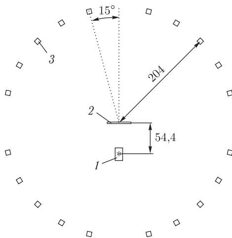
Рис. 20. Схема экспериментальной установки с пластиковыми сцинтилляционными детекторами: 1 — нейтронный генератор ИНГ-27; 2 — мишень; 3 — нейтронные детекторы, входящие в массив из 20 пластиковых сцинтилляционных детекторов. Все размеры приведены в миллиметрах
