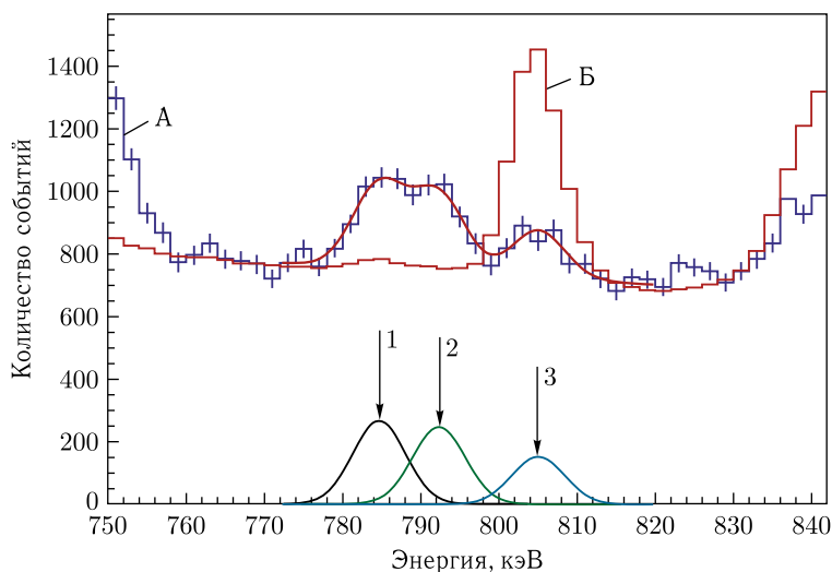
Рис. 14 (цветной в электронной версии). Пример аппроксимации \gamma -спектра, полученного с помощью ОЧГ-детектора при облучении образца из оксида хрома (синяя гистограмма, А), в сравнении со спектром антисовпадений (красная гистограмма, Б): 1 — пик 783,3 кэВ, реакция ^{50}\text{Cr}(n, n')^{50}\text{Cr} ; 2 — пик 791,3 кэВ, реакция ^{52}\text{Cr}(n, n')^{52}\text{Cr} ; 3 — фон
