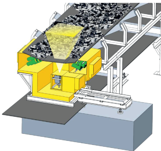
Рис. 33. Общая схема конвейерной установки АГП-К-1
