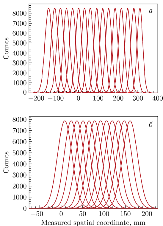
Рис. 9. Результаты аппроксимации гауссианами пространственных распределений 16 меченых пучков для \alpha -детектора с пикселями 4 (а) и 2 мм (б)
