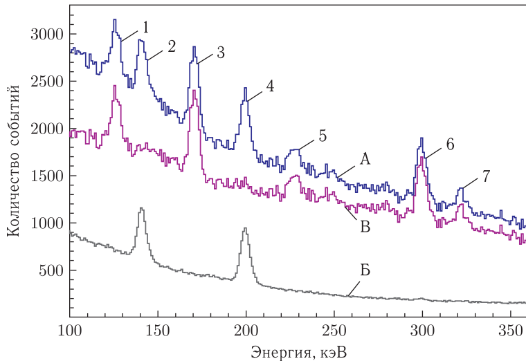
Рис. 13. Фрагмент энергетического спектра \gamma -квантов, измеренного ОЧГ-детектором для образца \text{Cg}_2\text{O}_3 : А — события в окне совпадений; Б — фон случайных совпадений в этом же окне; В — чистый спектр за вычетом фона случайных совпадений
