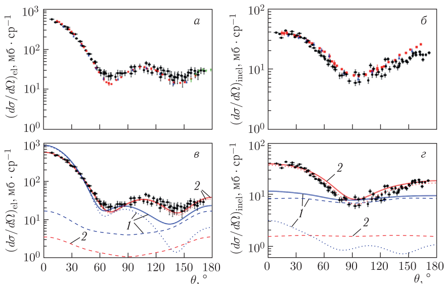
Рис. 22 (цветной в электронной версии). Полученные нами угловые распределения рассеянных нейтронов для основного состояния ( a, в ) и первого возбужденного состояния ядра ^{12}\text{C} ( б, з ) в сравнении с дифференциальными сечениями из других работ ( a, б ) и модельным расчетом TALYS 1.9 во вращательном приближении нулевой ( в, з ). Экспериментальные данные: черные кружки — наша работа; красные квадраты — [50]; синие треугольники — [51]; зеленые перевернутые треугольники — [52]. Результаты расчета в TALYS: синие линии (1) — с использованием параметров по умолчанию; красные линии (2) — с использованием параметров, полученных при аппроксимации наших данных; сплошная линия — дифференциальное сечение; пунктирная линия — вклад прямых процессов; штриховая линия — вклад процессов, идущих через составное ядро
