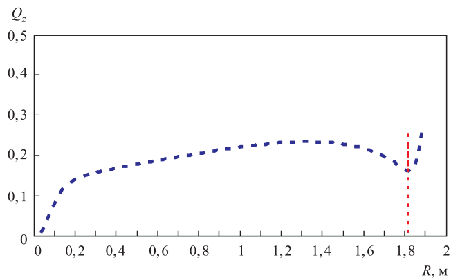
Рис. 11. Расчетные зависимости частоты аксиальных колебаний ( Q_z ) для энергии H^- 160 МэВ
