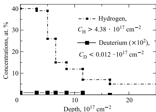
Рис. 5. Распределение водорода и дейтерия в 1 Nb-2-фольге
