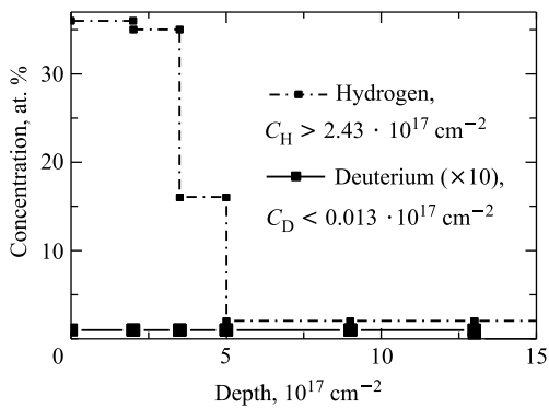
Рис. 3. Распределение водорода и дейтерия в ^1\text{Nb} -1-фольге
