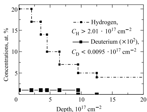
Рис. 8. Распределение водорода и дейтерия в Nb-3 2 -фольге
