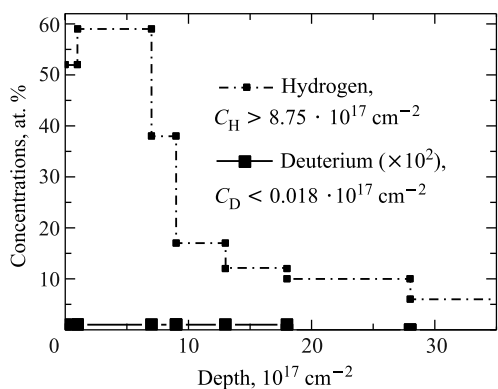
Рис. 7. Распределение водорода и дейтерия в 1 Nb-3-фольге
