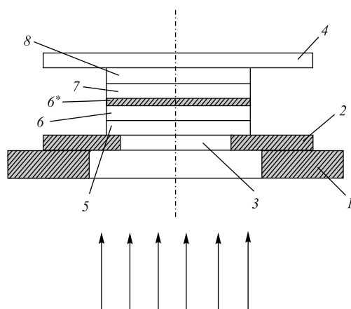
Рис. 1. Сборка Nb-фольг для изучения воздействия импульсов высокотемпературной плазмы на образцы на ПФ-4 [4, 5] (поток снизу): 1 — нижняя часть дискового держателя образцов на четыре сборки из нержавеющей стали X18H10T (НС); 2 — передняя диафрагма с диаметром отверстия 3, равным 10 или 15 мм; 4 — прижимная пластина из НС; 5–8 — набор фольг из одного или различных материалов. 6* означает, что фольга подвергнута с зачерненной стороны некоторой обработке
