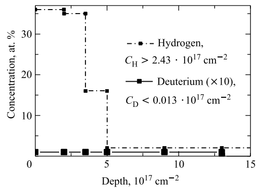
Рис. 4. Распределение водорода и дейтерия в Nb- 1^2 -фольге
