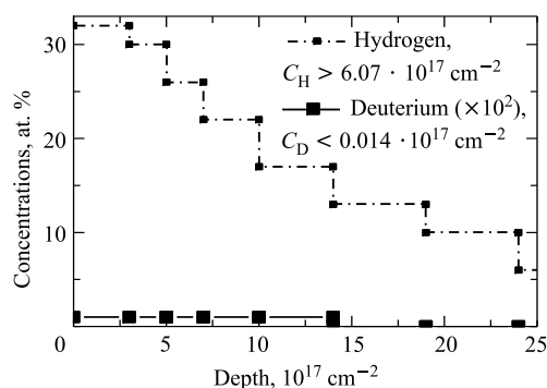
Рис. 6. Распределение водорода и дейтерия в Nb-2 2 -фольге
