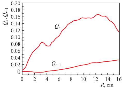
Fig. 6. Betatron tunes
