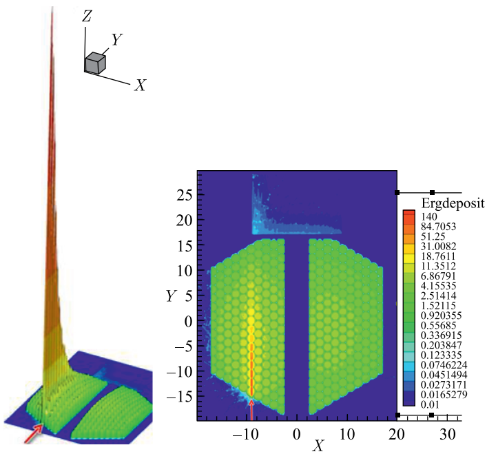
Рис. 17. Энерговывделение в АЗ и замедлителях, окружающих АЗ супербустера NEPTUN
