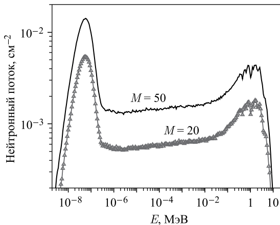
Рис. 11. Распределение потока тепловых нейтронов по энергии на поверхности плоского водяного замедлителя для двух значений умножения k_3 — 50 и 20
