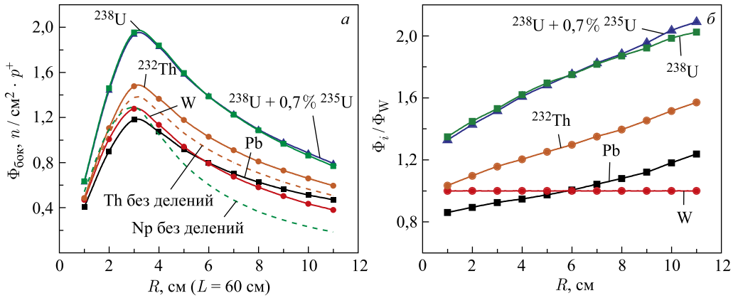
Рис. 2. Изменение средней плотности потока нейтронов на один протон с энергией 1 ГэВ на боковой поверхности цилиндрических мишеней длиной 60 см из вольфрама, свинца, тория, урана-238 и природного урана в зависимости от радиуса мишеней (а) и то же самое — относительно мишени из вольфрама (б)
