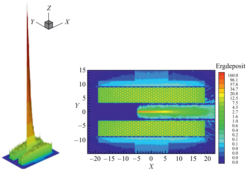
Рис. 16. Энерговывделение в мишени, АЗ и замедлителях, окружающих АЗ источника PLUTON
