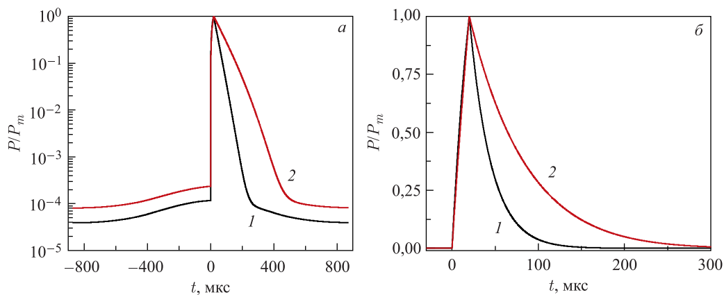
Рис. 7. Расчетная форма импульса мощности нейтронного источника в долях от максимального значения при K_{эф} = 0,98 для двух значений времени жизни мгновенных нейтронов — 0,5 (1) и 1,3 мкс (2); частота и длительность импульсов протонов составляет соответственно 30 Гц и 20 мкс: а) логарифмический масштаб, б) линейный
