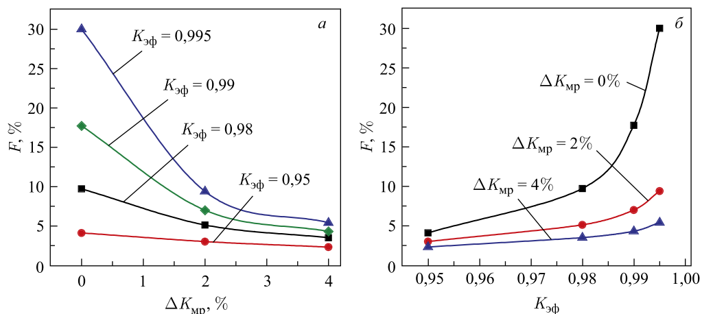
Рис. 5. Зависимость доли нейтронного фона между импульсами F от глубины модуляции реактивности \Delta K_{\text{мр}} при умножении 20 ( K_{\text{эф}} = 0,95 ), 50 ( K_{\text{эф}} = 0,98 ), 100 ( K_{\text{эф}} = 0,99 ) и 200 ( K_{\text{эф}} = 0,995 ) (а) и от K_{\text{эф}} при значениях \Delta K_{\text{мр}} = 0, 2 и 4\% (б). Время жизни мгновенных нейтронов \tau = 0,5 мкс
