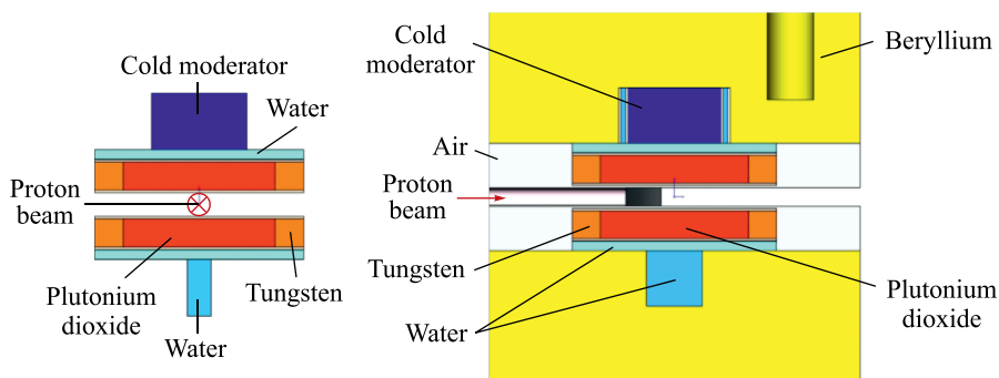
Рис. 6. Схема расчетной модели АЗ в окружении замедлителей
