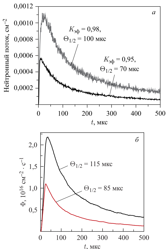
Рис. 8. Форма импульса тепловых нейтронов на поверхности плоского водяного замедлителя при значениях коэффициента размножения K_{эф} = 0,98 и 0,95 без модуляции реактивности: а) воздействие \delta -импульса протонов; б) импульс протонов длительностью 20 мкс
