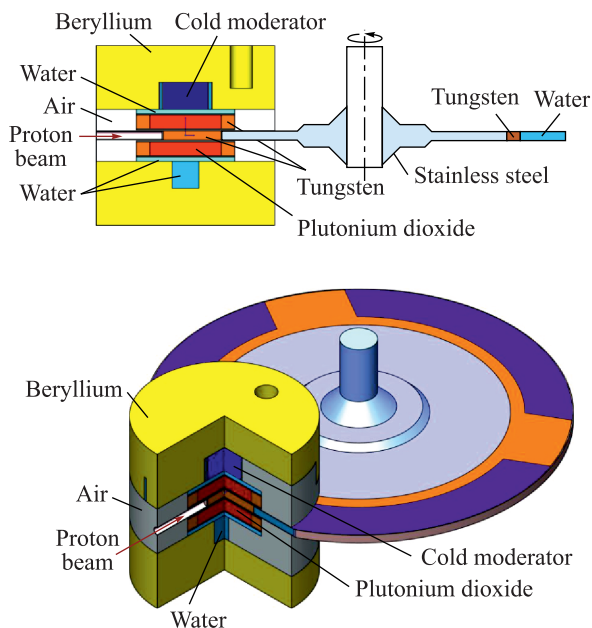
Рис. 1. Расчетная модель импульсного нейтронного источника с вращающейся вольфрамовой мишенью и АЗ из двуоксида плутония
