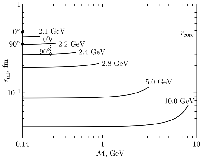
Рис. 2. Зависимость размера области взаимодействия от величины инвариантной массы рождаемой мезонной системы и энергии соударения. • — pp \rightarrow \{pp\}_s \pi^0 , \sqrt{s} = 2,2 ГэВ; о — pn \rightarrow d\pi^0\pi^0 , \sqrt{s} = 2,38 ГэВ. 0^\circ и 90^\circ обозначают угол вылета объединенной пары относительно оси реакции
