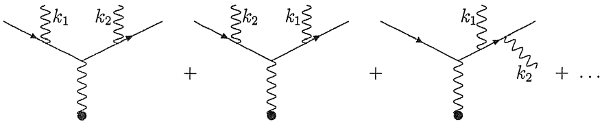
Рис. 1: Часть диаграмм Фейнмана, описывающих двойное тормозное излучение.
