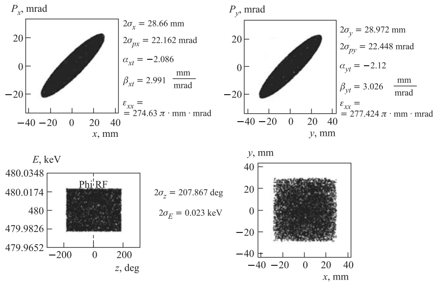
Рис. 3. Начальный эмиттанс из источника IS (см. рис. 1)
