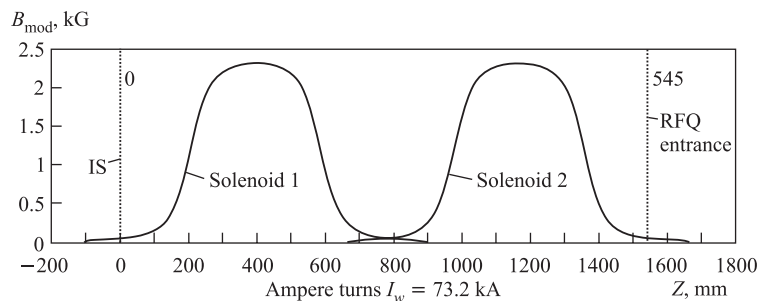
Рис. 2. Распределение магнитного поля вдоль осевой линии канала транспортировки
