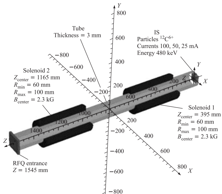
Рис. 1. Общий вид линии инжекции
