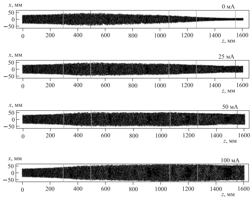
Рис. 4. Прохождение пучка через линию инжекции
