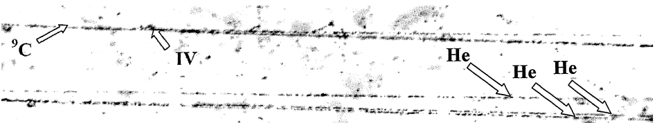
Рис. 13. Макрофотография «белой» звезды ^9\text{C} \rightarrow 3^3\text{He} при энергии 1.2 А ГэВ. На верхней фотографии видна вершина диссоциации (I.V.) и струя фрагментов в узком конусе; при продвижении вдоль струи различаются три релятивистских фрагмента (He) (нижняя фотография)
