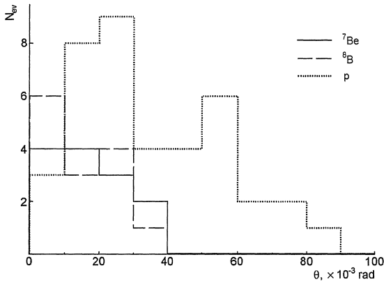
Рис. 7. Распределения по полярному углу \theta релятивистских фрагментов с зарядами в «белых» звездах \sum Z_{\text{fr}} = 5 + 1 и 4 + 1 + 1
