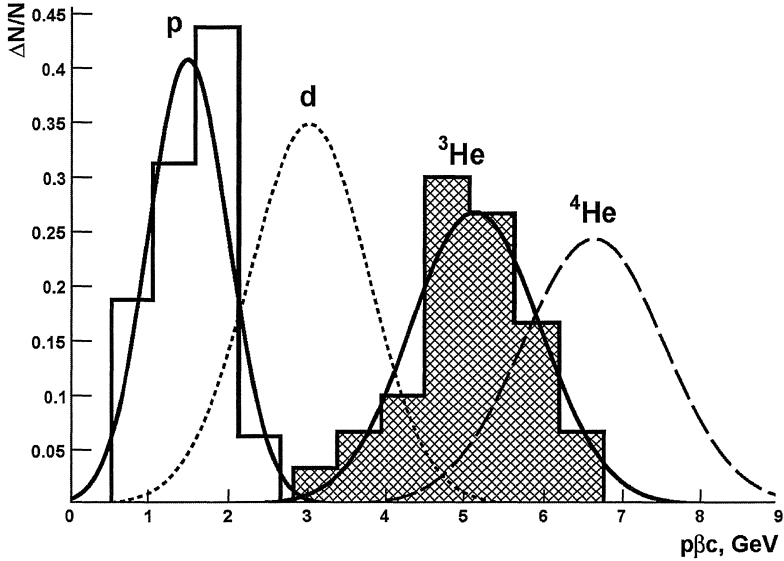
Рис. 2. Распределение измеренных величин r\beta c для следов ядер {}^3\text{He} из состава пучка ( {}^3\text{He} , заштрихованная гистограмма) и однозарядных фрагментов «белых» звезд ( \sum Z_{\text{fr}} = 5 + 1 + 4 + 1 + 1 ( p )) (открытая гистограмма); указаны ожидаемые распределения для дейтронов ( d ) и ядер {}^4\text{He}
