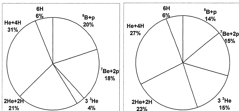
Рис. 4. Процентное соотношение основных каналов диссоциации ядра {}^9\text{C} в событиях с фрагментацией мишени (слева) и в «белых» звездах (справа)
