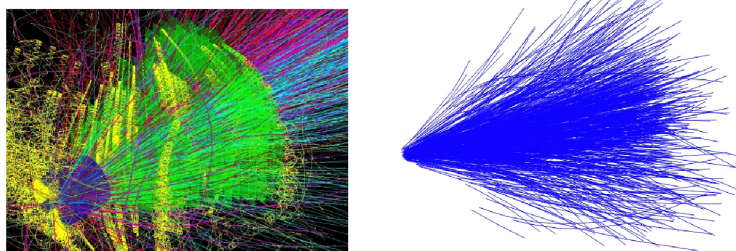
Рис. 2. Пример типичного для эксперимента CBM события, сгенерированного методом МК для центрального столкновения Au + Au при энергии 25 ГэВ/нуклон: слева — сгенерированное событие в MVD- и STS-детекторах, справа — реконструированное событие, содержащее 729 треков
