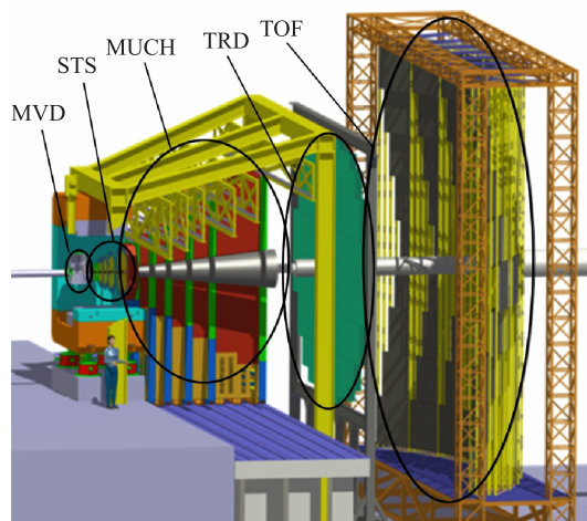
Рис. 1. Схема экспериментальной установки СВМ для регистрации мюонных распадов
