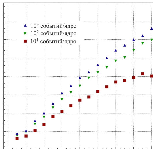
Рис. 10. Масштабируемость алгоритма распознавания треков для смешанных событий
