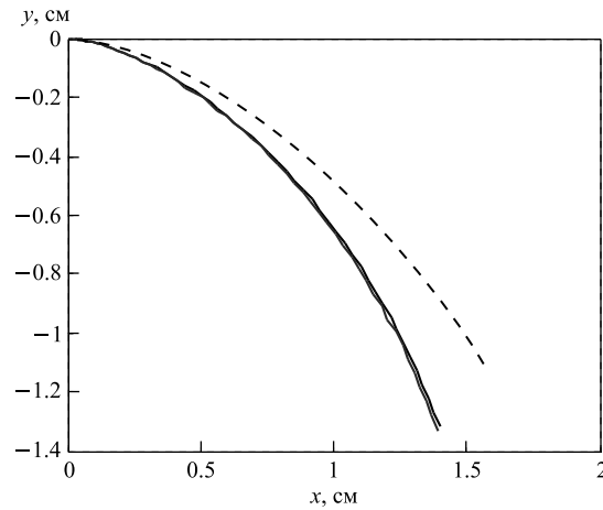
Рис. 6. Траектории иона \text{Kr}_{84}^{+11} с энергией 15 \text{ кэВ} \cdot Z в инфлекторе — штриховая линия, иона с энергией 10 \text{ кэВ} \cdot Z и проектного иона — сплошные линии
