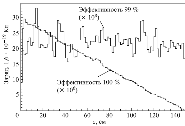
Рис. 4. Распределение пространственного заряда вдоль оси ТРС при эффективностях записания 99 и 100%
