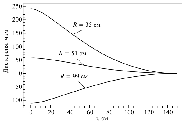
Рис. 6. Зависимость радиальной дистракции траекторий электронов при эффективности запыриания 100 % для различных значений радиуса
