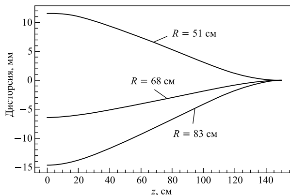
Рис. 7. Зависимость радиальной дисторсии траекторий электронов при эффективности запираения 99 % для различных значений радиуса
