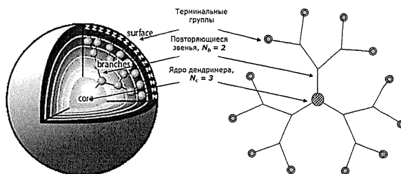
Рис. 1. Схематическое изображение дендримерной макромолекулы.
