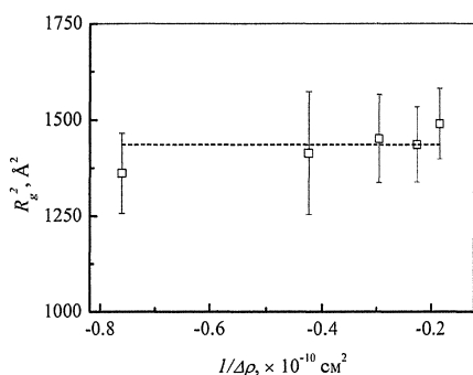
Рис. 6. Зависимость значения квадрата радиуса инерции R_g^2 от величины, обратной контрасту 1/\Delta\rho и его среднее значение, по данным малоуглового рассеяния на растворах полибутилкарбосилановых дендримеров девятой генерации.
