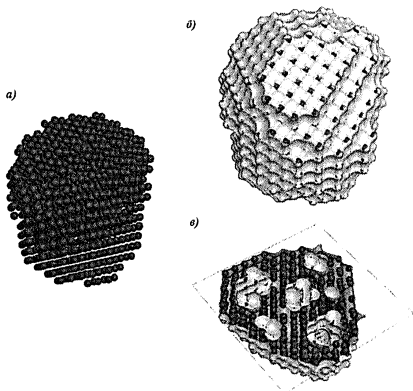
Рис. 12. а) – восстановленная модельная структура, состоящая из модельных атомов; б) – визуализация модели с использованием поверхности, получаемой на основании расчета методом Конолли; в) – сечение модели плоскостью.
