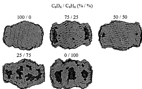
Рис. 7. Восстановленные модельные структуры в зависимости от степени дейтерирования растворителя. Представление в полупрозрачном виде. По данным малоуглового рассеяния на растворах полибутилкарбосилановых дендримеров девятой генерации.
