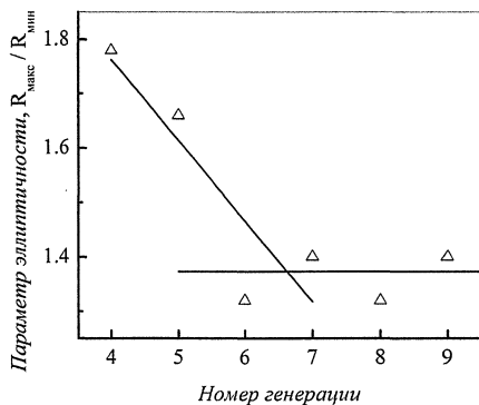
Рис. 2. Параметр эллиптичности моделей кремнийорганических дендримеров в зависимости от номера генерации. По данным малоуглового рассеяния нейтронов.
