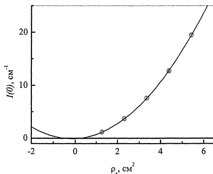
Рис. 5. Зависимость значения интенсивности рассеяния в нулевой угол I(0) от плотности амплитуды рассеяния растворителя \rho_s , по данным малоуглового рассеяния на растворах полибутилкарбосилановых дендримеров девятой генерации.
