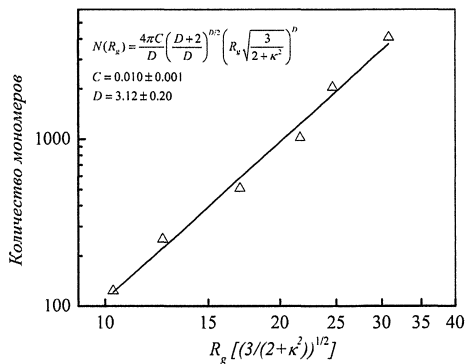
Рис. 3. Зависимость R_g от степени полимеризации N для анизотричной модели и ее аппроксимация функцией (3)
