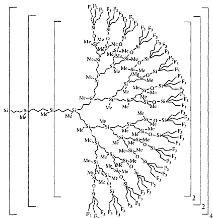
Рис. 8. Структурная формула кремнийорганического дендримера генерации 7.5 с фторуглеродными заместителями у атомов кремния во внешнем слое молекулярной структуры.
