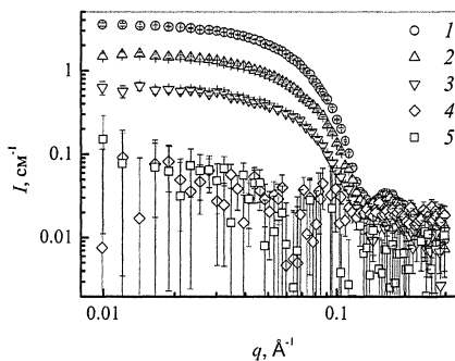
Рис. 9. Экспериментальные кривые малоуглового рассеяния нейтронов на растворах кремнийорганических дендримеров G7.5(F): Ацетон-д 6 /Ацетон (%/%) 1 - 100/0, 2 - 75/25, 3 - 50/50, 4 - 25/75, 5 - 0/100.
