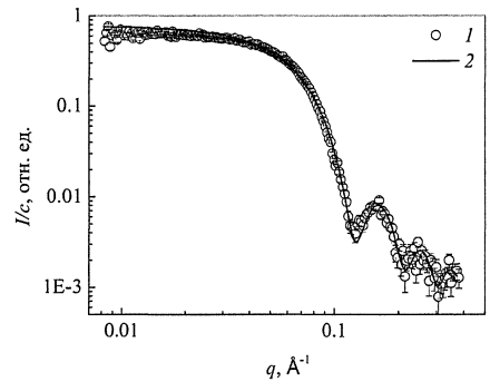
Рис. 11. 1 - Кривая малоуглового рассеяния, полученная линейной экстраполяцией кривых к бесконечному разбавлению, в области малых векторов рассеяния, отвечающих разным концентрациям суспензий дендримеров; 2 – восстановленная функция интенсивности рассеяния I(q) по найденной функции p(r) .
