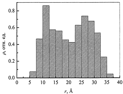
Рис. 13. Радиальная функция распределения плотности \rho(r) в модели.
