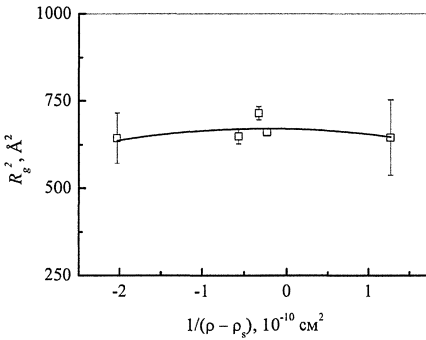
Рис. 10. Зависимость значения квадрата радиуса инерции R_g^2 от величины, обратной контрасту 1/\Delta\rho и аппроксимация функцией параболы, по данным малоуглового рассеяния нейтронов на растворах карбосилановых дендримеров генерации 7.5 с фторуглеродными заместителями у атомов кремния во внешнем слое молекулярной структуры.
