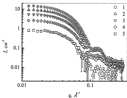
Рис. 4. Экспериментальные кривые малоуглового рассеяния нейтронов на растворах полибутилкарбосилановых дендримеров девятой генерации: C 6 D 6 /C 6 H 6 (%/%) 1 - 100/0, 2 - 75/25, 3 - 50/50, 4 - 25/75, 5 - 0/100.
