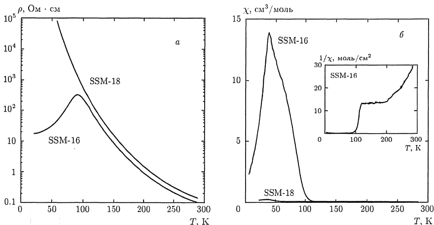
Рис. 2. Температурные зависимости электрического сопротивления (а) и магнитной восприимчивости (б) для \text{Sm}_{0,5}\text{Sr}_{0,5}\text{MnO}_3 (SSM) с ^{16}\text{O} и ^{18}\text{O} изотопами. Зависимость 1/\chi(T) для SSM-16 показана на вставке [7].
