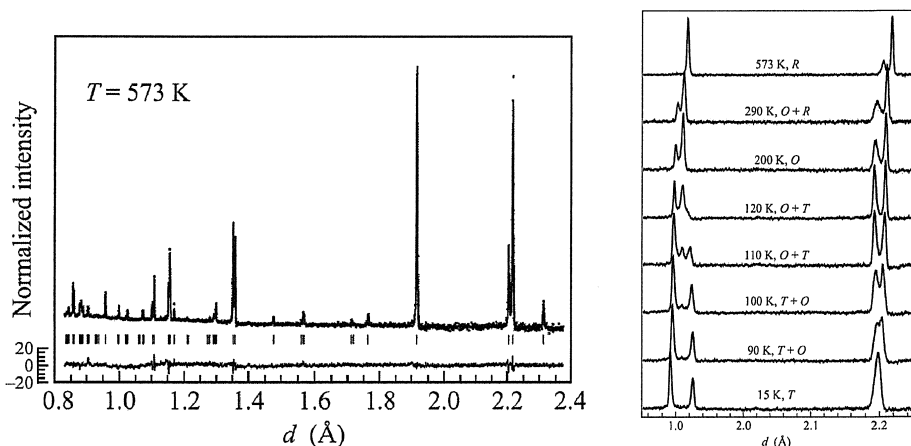
Рис. 7. Слева нейтронный дифракционный спектр \text{Pr}_{0.5}\text{Sr}_{0.5}\text{CoO}_3 , измеренный на ФДВР/ИБР-2 при T = 573 К и обработанный по методу Ритвельда. Вертикальные штрихи указывают рассчитанные положения дифракционных пиков в фазе R\bar{3}c . Разностная кривая нормирована на стандартное отклонение в точке. Справа участок дифракционного спектра PSCO, измеренного при различных температурах. На картинке обозначены температура (от 15 до 573 К) и структурные фазы ( R = R\bar{3}c , O = Imma , T = I-1 ).
