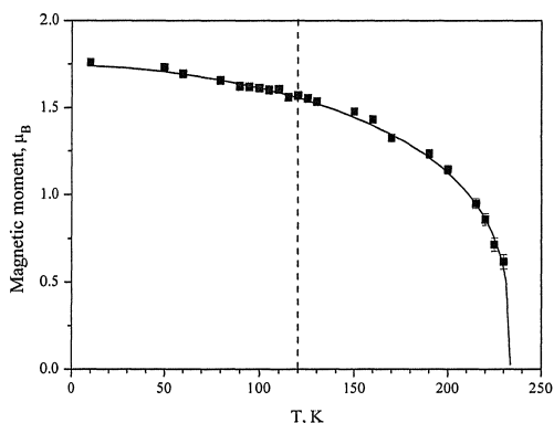
Рис. 10. Зависимость от температуры среднего (для двух фаз) упорядоченного магнитного момента кобальта и ее описание феноменологической формулой \mu(T) = \mu(0)[1 - (T/T_C)^q]^\beta с параметрами: \mu(0) = 1.74 \mu_B , T_C = 233.8 К, q = 1.79 , \beta = 0.31 .
