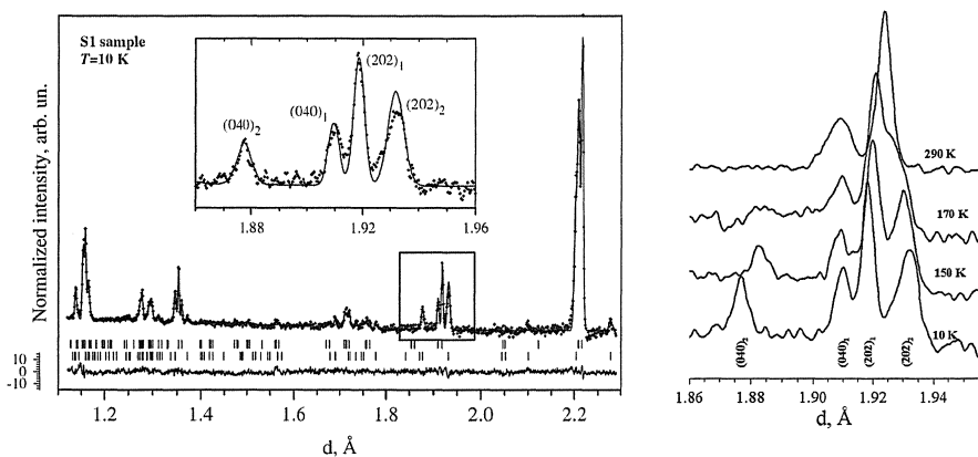
Рис. 5. Слева дифракционный спектр NTSM-S1, измеренный на ФДВР/ИБР-2 при T=10 К и обработанный по методу Ритвельда. Вертикальные штрихи указывают рассчитанные положения дифракционных пиков двух структурных фаз. На вкладке показан участок дифракционного спектра, на котором четко виден вклад двух структурных фаз. Справа эволюция участка дифракционного спектра NTSM-S1, отображенного на вкладке левого рисунка, при переходе от одно - к двухфазному состоянию и видно появление новой структурной фазы при понижении температуры. Указаны индексы Миллера с принадлежностью к первой и ко второй фазе.
