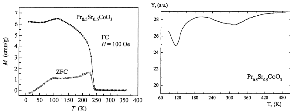
Рис. 3. Слева зависимость намагниченности PSCO от температуры. При T \approx 120 К видно аномальное поведение кривой намагниченности [9]. Справа зависимость Модуля Юнга для PSCO от температуры [9]. Аномалии упругих свойств совпадают с магнитными аномалиями.
