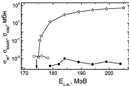
Рис. 4: Зависимость полных сечений образования остатков испарения в реакциях ^{100}\text{Mo} + ^{100}\text{Mo} \rightarrow ^{200}\text{Po} , ^{100}\text{Mo} + ^{110}\text{Pd} \rightarrow ^{210}\text{Ra} , ^{110}\text{Pd} + ^{110}\text{Pd} \rightarrow ^{220}\text{U} (а) и ^{16}\text{O} + ^{208}\text{Pb} \rightarrow ^{224}\text{Th} (б) от энергии реакции ( E_{c.m.} ). Точки: \circ — на первой стадии расчета ядра ориентированны “нос к носу”; \bullet — случайная ориентация; стрелки — рассчитанные нами барьеры реакций; звездочки — экспериментальные данные; точечные линии — результаты расчета в модели конкуренции каналов полного слияния и квазиделения в симметричных ядерных реакциях; перечеркнутые квадраты ([7]), круги ([8]) и треугольники ([9]) — экспериментальные данные.
