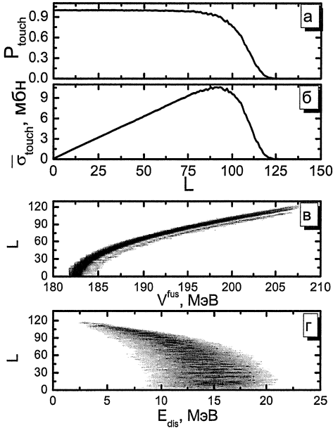
Рис. 3: Характеристики системы в точке касания в реакции ^{100}\text{Mo} + ^{100}\text{Mo} \rightarrow ^{200}\text{Po} ( E_{\text{c.m.}} = 215 МэВ): панели a и b — зависимости вероятности касания и частичного сечения касания от углового момента системы; панель v — распределение событий касания по потенциальной энергии системы и ее угловому моменту в точке касания; панель z — распределение событий касания по внутренней энергии и ее угловому моменту.
