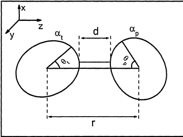
Рис. 1: Вид системы на первой стадии расчета. Форма системы описывается следующими параметрами: параметрами деформации ядра “мишени” \alpha_t и ядра “снаряда” \alpha_p ; углами \theta_t и \theta_p , описывающими отклонение осей симметрии ядер от линии, соединяющей их центры масс; величиной r , задающей расстояние между центрами масс ядер. Величина d характеризует расстояние между ближайшими точками поверхностей ядер. Оси симметрии ядер и линия, соединяющая их центры масс, лежат в плоскости XOZ .
