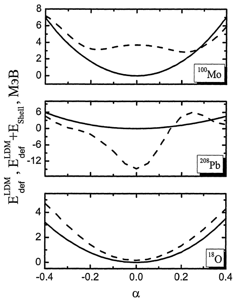
Рис. 2: Зависимость потенциальной энергии ядер ^{100}\text{Mo} , ^{208}\text{Pb} и ^{18}\text{O} от деформации с учетом ( E_{\text{def}}^{\text{LDM}} + E_{\text{shell}} ) (штриховая кривая) и без учета ( E_{\text{def}}^{\text{LDM}} ) (сплошная кривая) оболочечных поправок. Учет ОС может приводить к изменению формы ядер в основном состоянии ( ^{100}\text{Mo} ) и к изменению жесткости потенциала ( ^{208}\text{Pb} и ^{18}\text{O} ).
