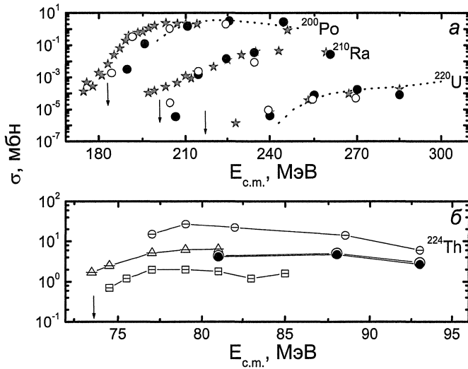
Рис. 4: Зависимость полных сечений образования остатков испарения в реакциях ^{100}\text{Mo} + ^{100}\text{Mo} \rightarrow ^{200}\text{Po} , ^{100}\text{Mo} + ^{110}\text{Pd} \rightarrow ^{210}\text{Ra} , ^{110}\text{Pd} + ^{110}\text{Pd} \rightarrow ^{220}\text{U} (а) и ^{16}\text{O} + ^{208}\text{Pb} \rightarrow ^{224}\text{Th} (б) от энергии реакции ( E_{c.m.} ). Точки: \circ — на первой стадии расчета ядра ориентированны “нос к носу”; \bullet — случайная ориентация; стрелки — рассчитанные нами барьеры реакций; звездочки — экспериментальные данные; точечные линии — результаты расчета в модели конкуренции каналов полного слияния и квазиделения в симметричных ядерных реакциях; перечеркнутые квадраты ([7]), круги ([8]) и треугольники ([9]) — экспериментальные данные.
