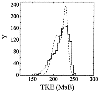
Рис. 7: Рассчитанное (пунктирные линии) распределение кинетической энергии (верхняя часть) и массовое распределение (нижняя часть) фрагментов деления ^{258}\text{Fm} в сравнении с экспериментальными данными (гистограмма).
