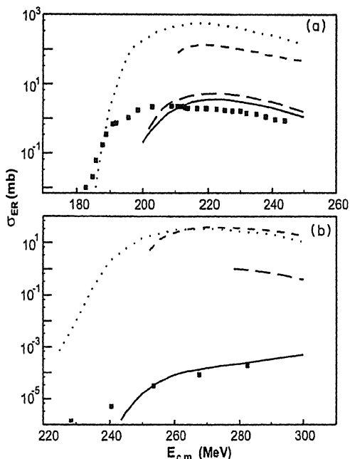
Рис. 1: Зависимость сечений образования испарительных остатков от энергии E_{c.m.} для реакций ^{100}\text{Mo} + ^{100}\text{Mo} (а) и ^{110}\text{Pd} + ^{110}\text{Pd} (б). Результаты расчетов в рамках оптической модели, модели поверхностного трения, динамической макроскопической модели и нашей модели показаны пунктирной линией, короткими штрихами, длинными штрихами и сплошной линией соответственно. Экспериментальные данные показаны квадратами.
