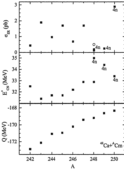
Рис. 6: Максимумы функций возбуждения в канале 3n (вверху) при соответствующих энергиях возбуждения составного ядра (середина) и значения Q (внизу) для реакций слияния ^{48}\text{Ca} + ^A\text{Cm} (темные символы) как функции A . Отмечены максимальные сечения образования испарительных остатков в канале 4n. Экспериментальные данные для реакции ^{48}\text{Ca} + ^{248}\text{Cm} \rightarrow ^{292}116 + 4n ( E_{CN}^* \approx 31 - 36 MeV) показаны светлым кружком.
