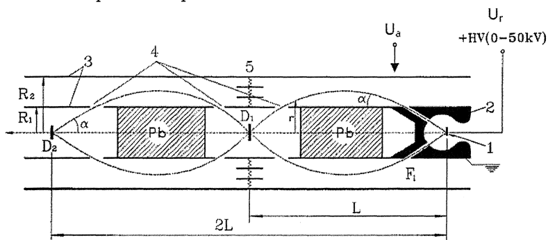
Рис. 1. Принципиальная схема электростатического спектрометра ESA-50: 1 - радиоактивный источник (внутренняя сфера замедлителя); 2 - внешняя сфера замедлителя; F_1 - коническая диафрагма; 3 - внешний и внутренний цилиндры; 4 - круговые диафрагмы; 5 - изоляторы с промежуточными цилиндрами.
