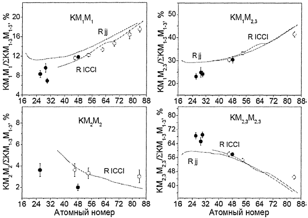
Рис. 9. Зависимость относительных интенсивностей KM_1M_1 , KM_1M_{2,3} и KM_{2,3}M_{2,3} переходов от атомного номера Z . Сплошные линии – релятивистские расчеты в схеме jj (R jj ) и промежуточной связи (R ICCI) с учетом взаимодействия конфигураций; темные кружки – результаты наших измерений; светлые кружки – литературные данные.
