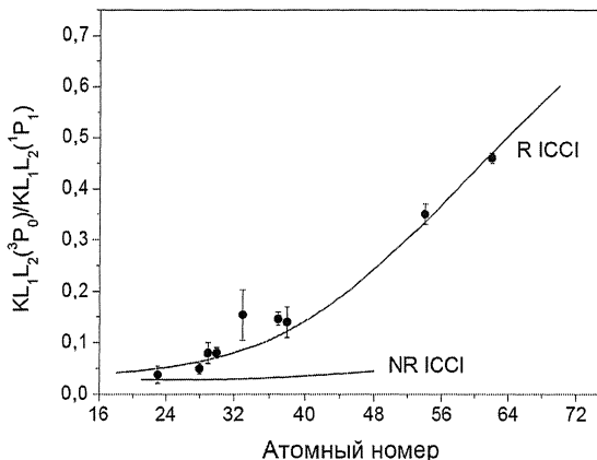
Рис. 7. Зависимость распределения интенсивности в пределах дублета KL_1L_2(^1P_1, ^3P_0) от Z . Сплошные линии – релятивистские (R ICCI) и нерелятивистские (NR ICCI) расчеты в схеме промежуточной связи с учетом взаимодействия конфигураций. Темные кружки – результаты наших измерений.
