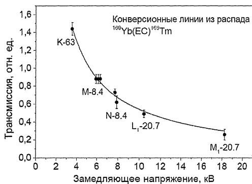
Рис. 3. Зависимость трансмиссии спектрометра ESA-50 от замедляющего напряжения U ( \Delta E_{инст} \sim 7 эВ). Сплошная линия - результат фитирования данных функцией U_0/U .
