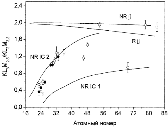
Рис. 8 Зависимость отношения интенсивностей KL_3M_{2,3} и KL_2M_{2,3} переходов от атомного номера Z . Сплошные линии – релятивистские (R jj ) и нерелятивистские расчеты в схеме jj (NR jj ) и промежуточной связи (NR IC1), (NR IC2); темные кружки – наши данные; светлые кружки – данные других экспериментов.
