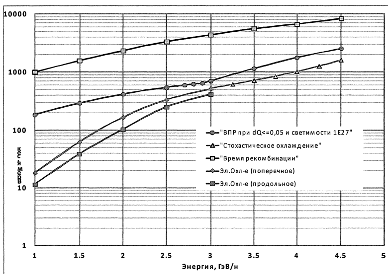
Рис. 3. Характерные времена нагрева за счет внутривидового рассеяния для устойчивой динамики ионного пучка, характерные времена электронного охлаждения для энергии ионов до 3 ГэВ/н в режиме ДПЗ, и стохастического охлаждения для энергии выше 3 ГэВ/н для полосы частот 3-6 ГГц.
