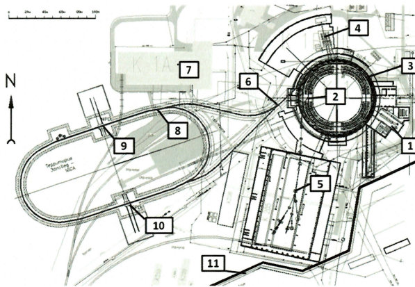
Рис. 1. Схема комплекса NICA. 1 - инжектор, 2 – Бустер, 3 - Нуклотрон, 4 – гелиевый ожижительный комплекс, 5 – экспериментальный корпус для установок на выведенных пучках, 6 - каналы транспортировки пучка в коллайдер, 7 – системы питания всего комплекса, 8 – Коллайдер; 9 и 10 – детекторные установки MPD и SPD, 11 – периметр площадки ЛФВЭ ОИЯИ.
