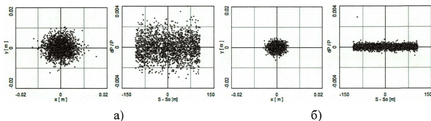
Рис.2. Результаты моделирования эволюции параметров пучка ионов ^{197}\text{Au}^{32+} на энергии 3 МэВ/н: распределение частиц на фазовых плоскостях (x, x') и (x, dp/p) до (а) и после охлаждения (б).
