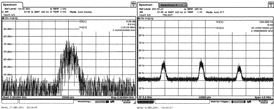
Рис. 5. Примеры экспериментально измеренных спектров шума пучка на энергии 2 ГэВ/н. Слева - пучок дейтронов, справа - пучок ионов C^{6+} .
