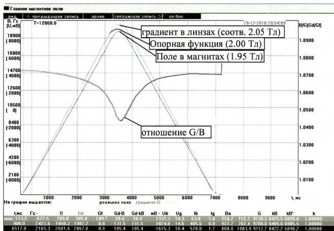
Рис. 4. Диаграмма цикла с полем дипольных магнитов на столе 2 Тл. Отношение G/B – отношение градиента линз к полю дипольных магнитов.
