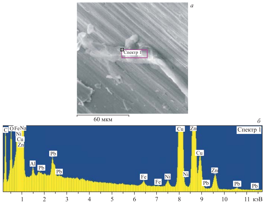
Рис. 21. СЭМ-изображение структуры на поверхности ЛВ (а) и ХСРИ (б)
