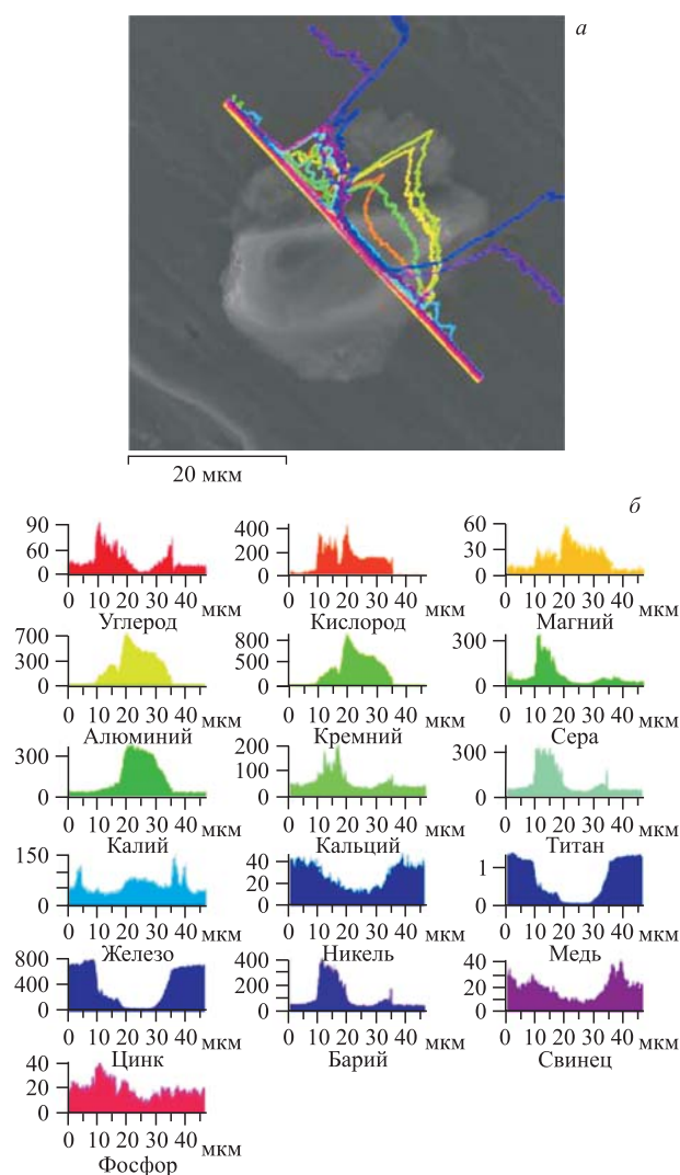
Рис. 18. СЭМ-изображение структур на поверхности ЛВ, вдоль выделенной полосы на котором выполнен РМЗА (а), и соответствующие распределения (б)
