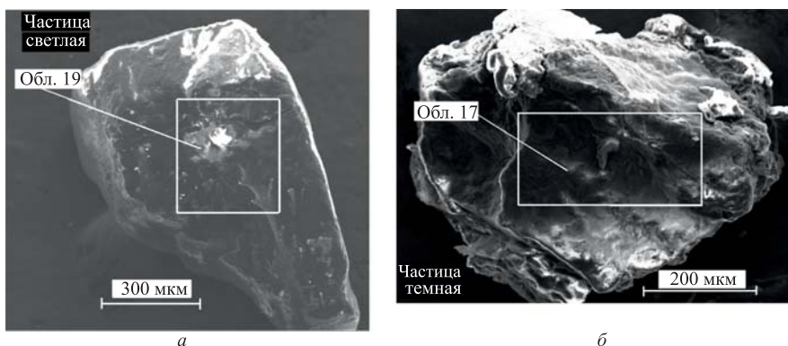
Рис. 4. СЭМ-изображения светлой (а) и темной (б) частиц в обл. 19 и 17, где были сделаны РМЗА
