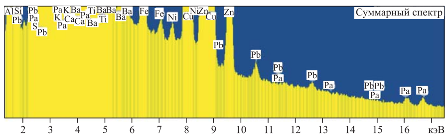
Рис. 19. Суммарный ХСРИ, соответствующий РМЗА по полосе на рис. 18 а
