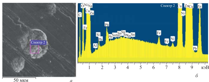
Рис. 6. СЭМ-изображение структуры на поверхности ЛВ ( а ) и ХСРИ ( б )
