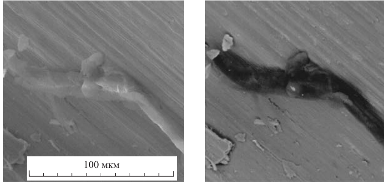
Рис. 20. СЭМ-изображение разветвленной структуры на поверхности ЛВ, слева во вторичных, а справа в отраженных электронах
