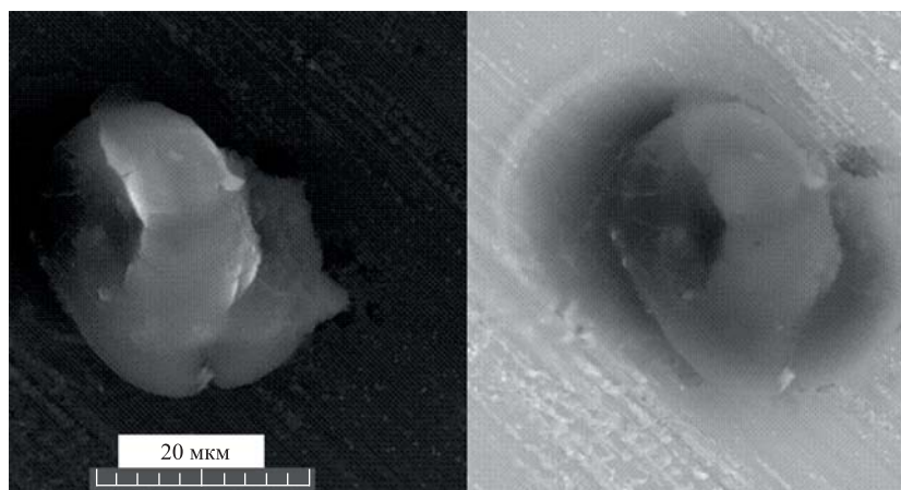
Рис. 15. СЭМ-изображение структуры в виде «тора» слева во вторичных, а справа в отраженных электронах
