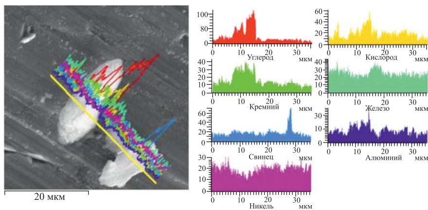
Рис. 10. СЭМ-изображение двух структур на поверхности ЛВ, вдоль выделенной полосы на котором выполнен РМЗА ( а ), и соответствующие распределения ( б )
