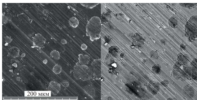
Рис. 12. СЭМ-изображение внутренней поверхности ЛВ
