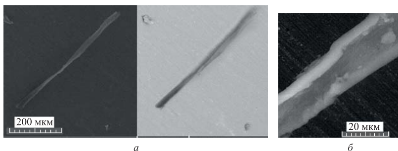
Рис. 13. СЭМ-изображение длинной структуры в виде половинки трубки (а), слева во вторичных, а справа в отраженных электронах, и увеличенное изображение этой структуры (б)
