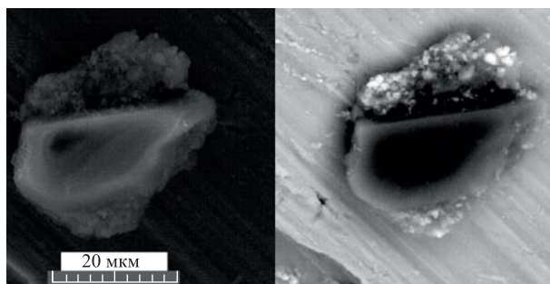
Рис. 17. СЭМ-изображение структуры в виде плотной частицы и более мелких вкраплений, слева во вторичных, а справа в отраженных электронах
