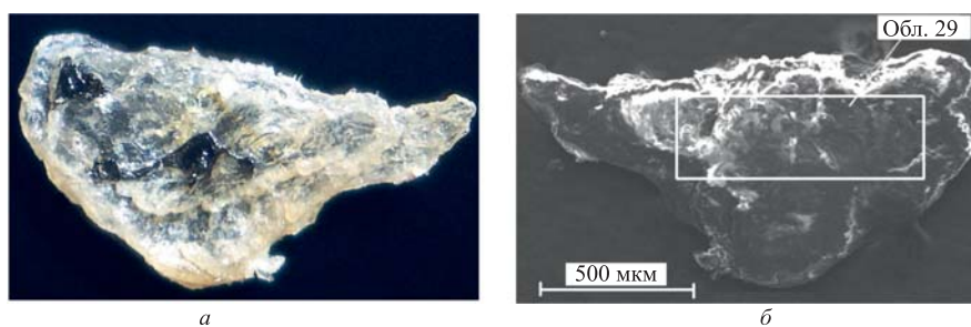
Рис. 1. Фотография синтезированной частицы с размерами 1,5 мм на 0,75 мм ( а ) и СЭМ-изображение синтезированной частицы, в обл. 29 которого сделан РМЗА ( б )
