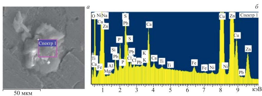
Рис. 5. СЭМ-изображение структуры на поверхности ЛВ ( а ) и ХСРИ ( б )
