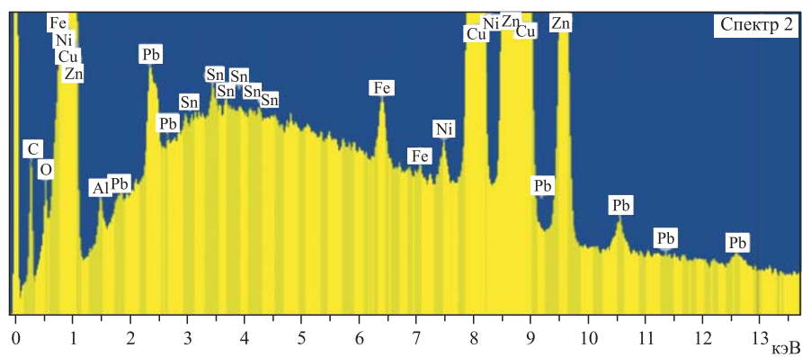
Рис. 22. ХСРИ, измеренный на срезе латунной втулки
