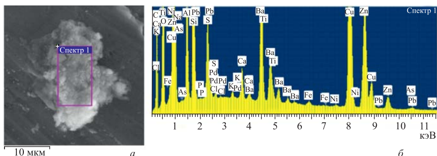
Рис. 7. СЭМ-изображение структуры на поверхности ЛВ (а) и ХСРИ (б)
