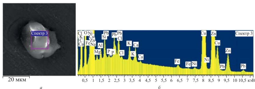
Рис. 16. СЭМ-изображение структуры на поверхности ЛВ (а) и ХСРИ (б)
