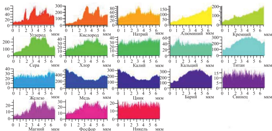
Рис. 9. Распределения элементов, полученные при проведении РМЗА при сканировании по полосе вдоль наиболее рыхлой части структуры
