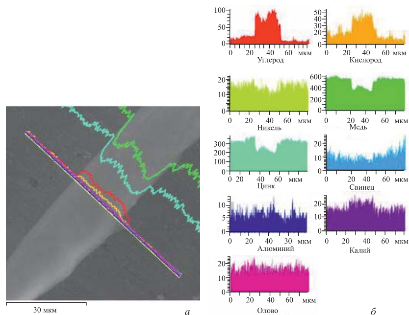
Рис. 14. СЭМ-изображение структур на поверхности ЛВ, вдоль выделенной полосы на котором выполнен РМЗА ( а ), и соответствующие распределения ( б )
