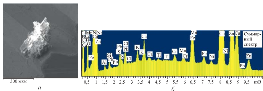
Рис. 11. СЭМ-изображение структуры на поверхности ЛВ (а) и ХСРИ (б)
